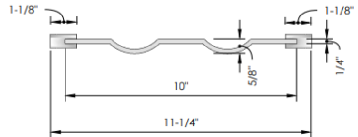
Elevation B
